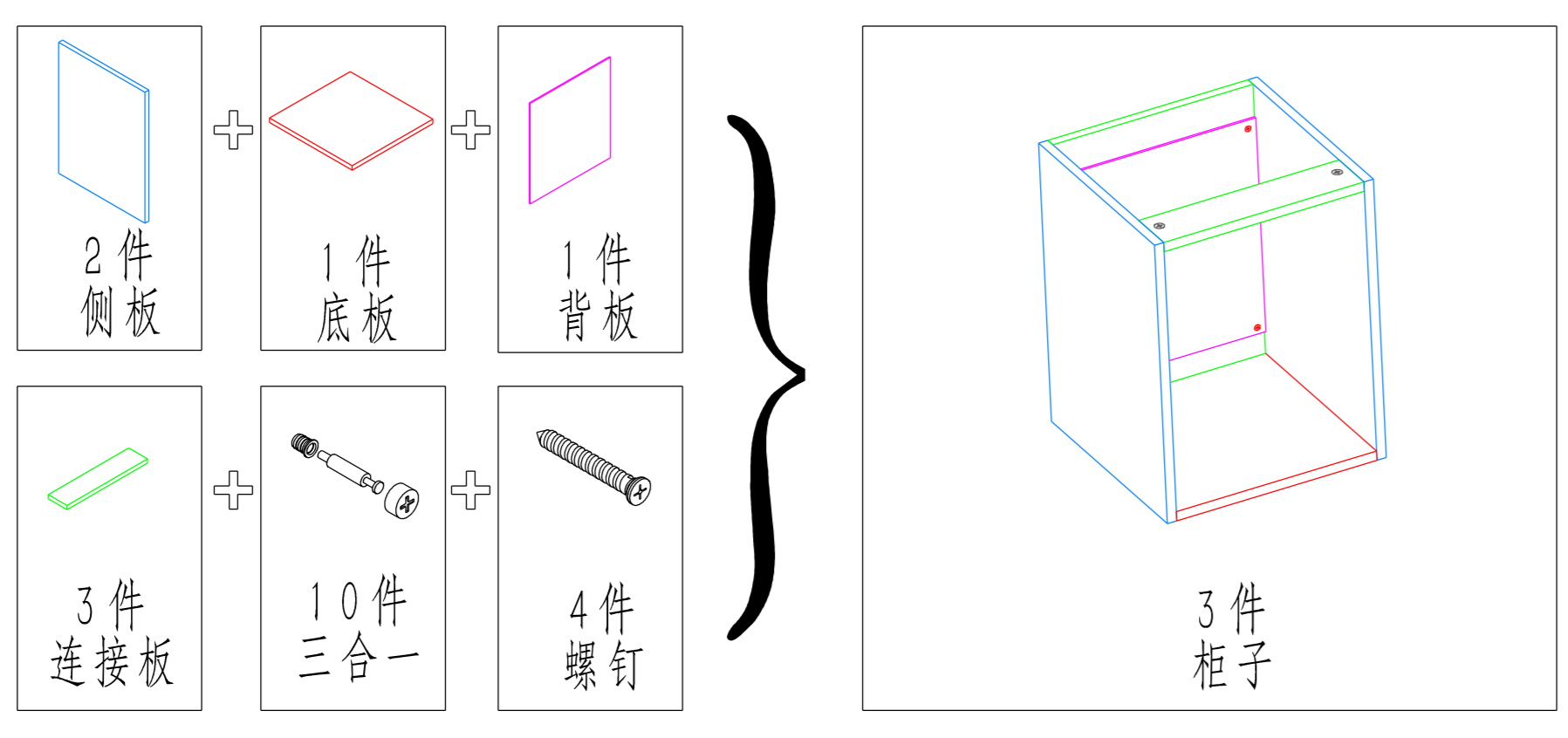
柜子的安装图示:
